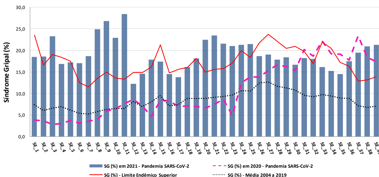
Figura 20 – Diagrama de controle da proporção de Síndrome Gripal (SG) por SE de início de sintomas, RS, 2021
